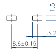
P.C.B. LAYOUT
