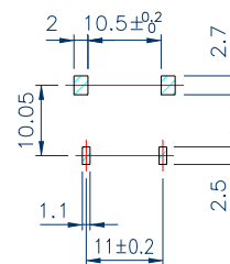
P.C.B. LAYOUT
