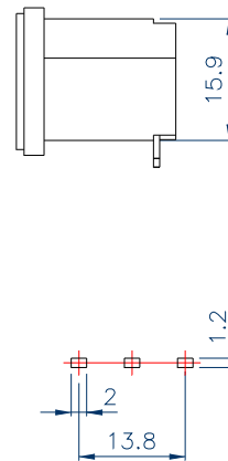
P.C.B. LAYOUT
